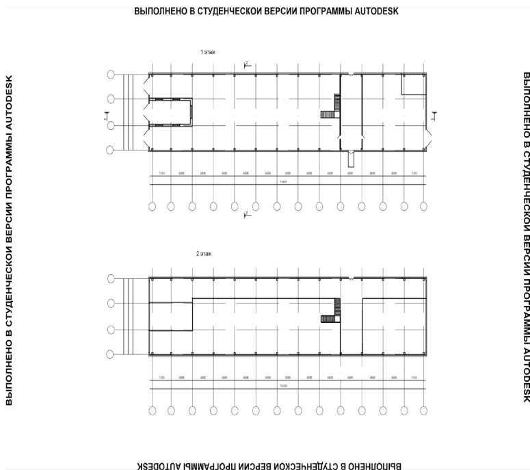
ВЫПОЛНЕНО В СТУДЕНЧЕСКОЙ ВЕРСИИ ПРОГРАММЫ AUTODESK Рис. 5. Поэтажные планы сооружения
